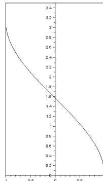
Arccosinus
