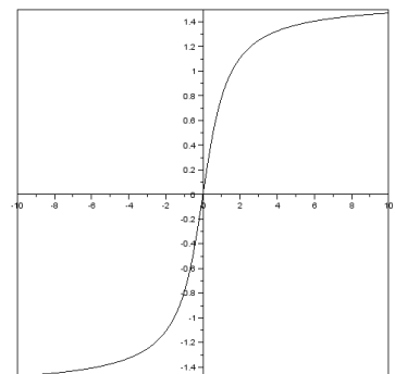
Arctangente
